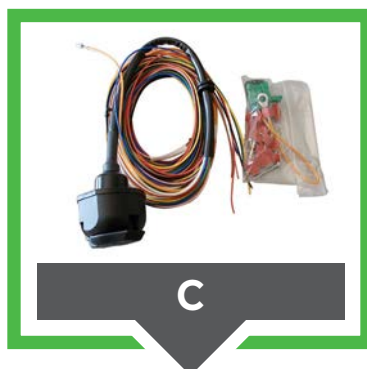
Cablaggio elettrico semplice a 13 poli senza centralina
